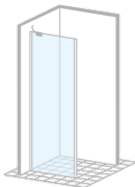
Элемент В* Боковая стенка 90/100/120 x 200 см W30G-W90-200-CT L/R W30G-W100-200-CT-R W30G-W120-200-CT L/R
