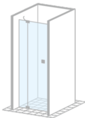
Элемент А* Душевая дверь в нишу с неподвижным элементом 80/90/100/120 x 200 см W30G-E3D5-200-CT-L/R W30G-E3D6-200-CT-L/R W30G-E3D7-200-CT-L/R W30G-E3D9-200-CT-L/R
